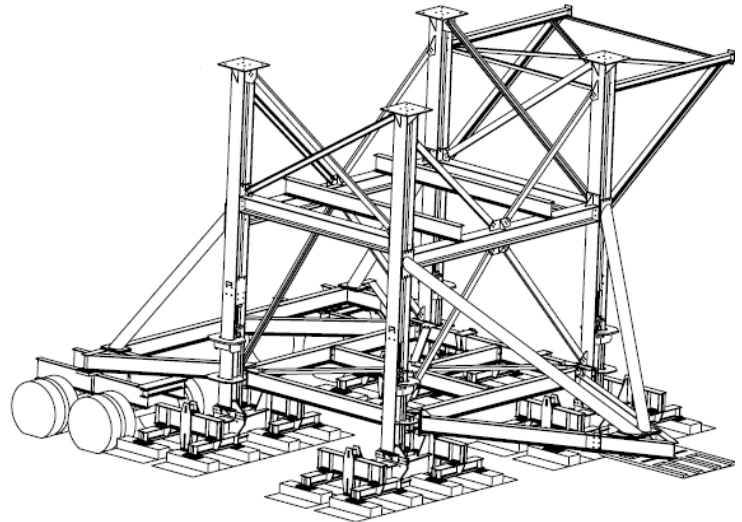
ESTRUCTURA TOLVA MOVIL PUERTO BURDEOS. FRANCIA
