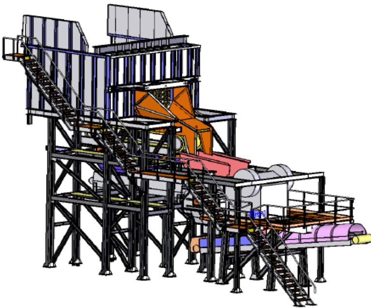
PUESTO PRIMARIO PLANTA ARIDOS. GUINEA BISSAU
