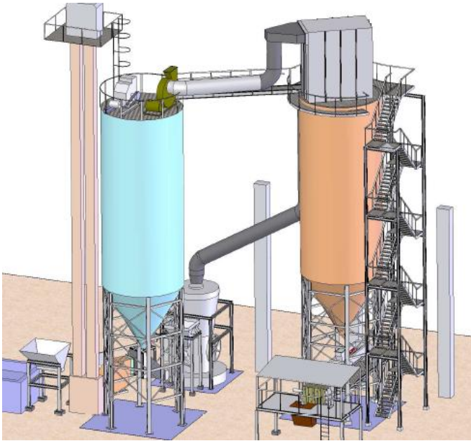
SILOS DE DOLOMITA Y NITRATO. PLANTA FERTILIZACION. ARGELIA
